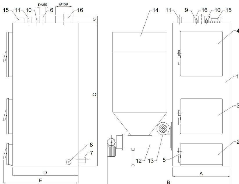
Rys.1. Kocioł „EKO 5S”
